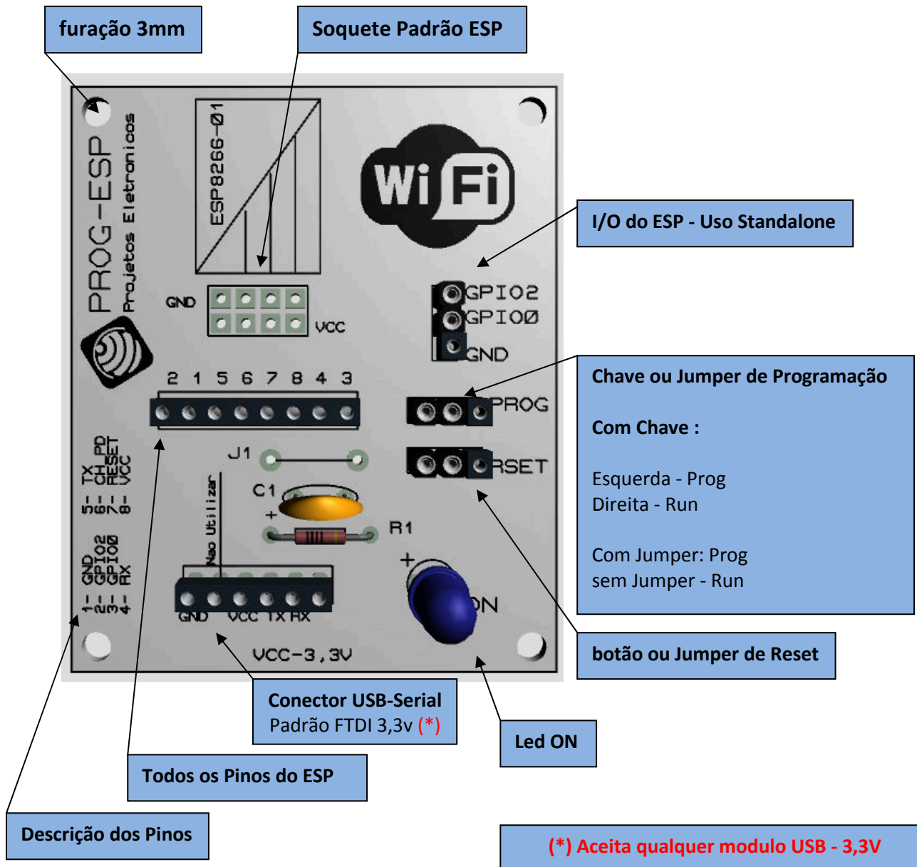
Descrição de todos os componentes da placa
