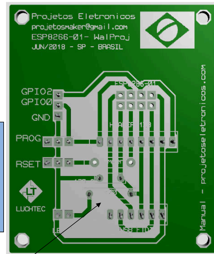
Descrição de todos os componentes da placa
